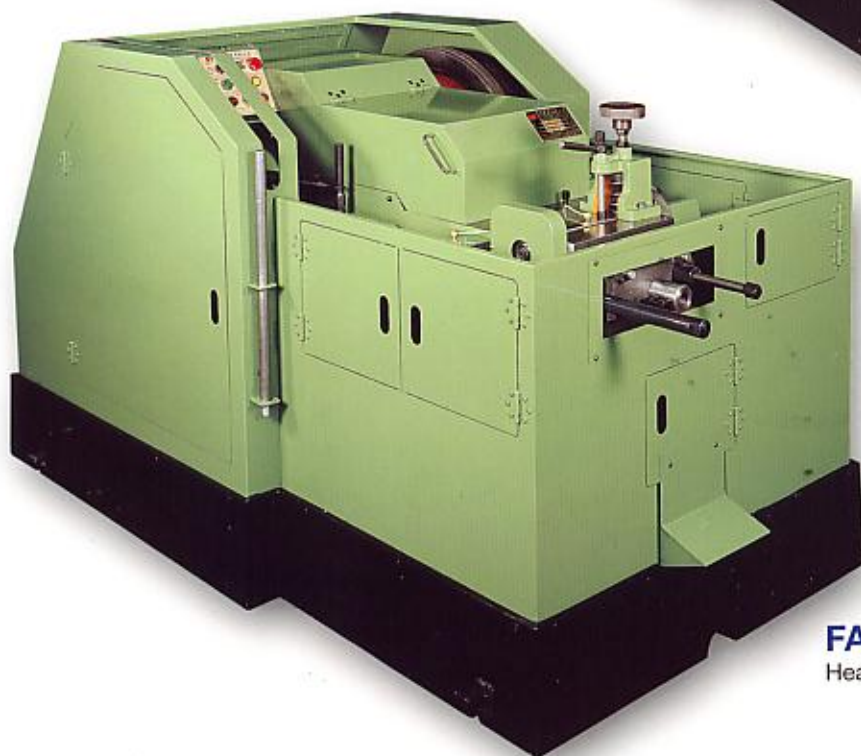
半密封打頭機 Heading Machine & Semi-Cover
