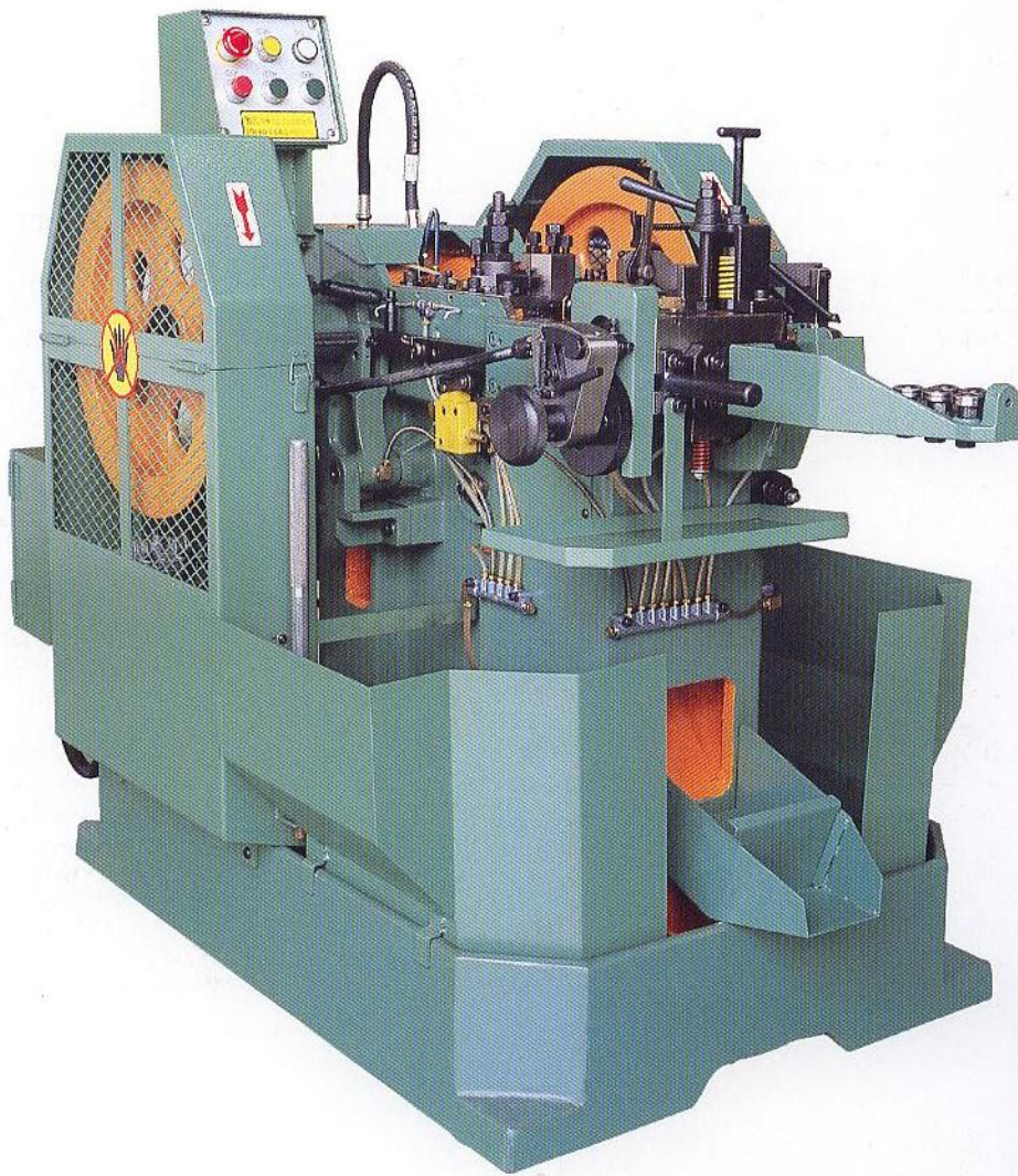
HC-3HB 高速冷鍛螺絲打頭機 High Speed Heading Machine
